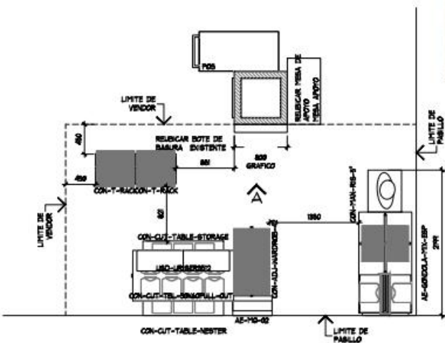
PLANTA DE MOBILIARIO ESC. 1:50
