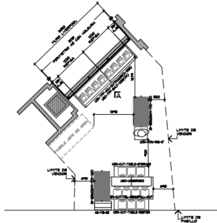
PLANTA ARQUITECTONICA ESC. 1:50
