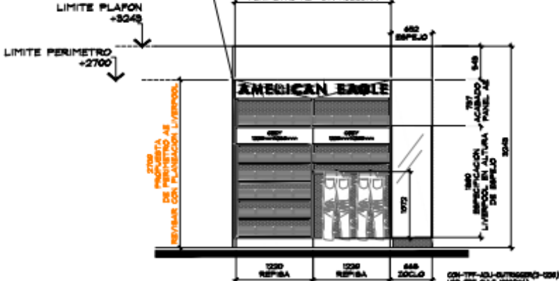
ALZADO "B" ESC. 1:50
