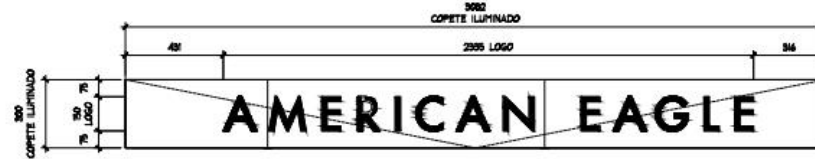
DETALLE DE LETRERO A ESC. 1:20
