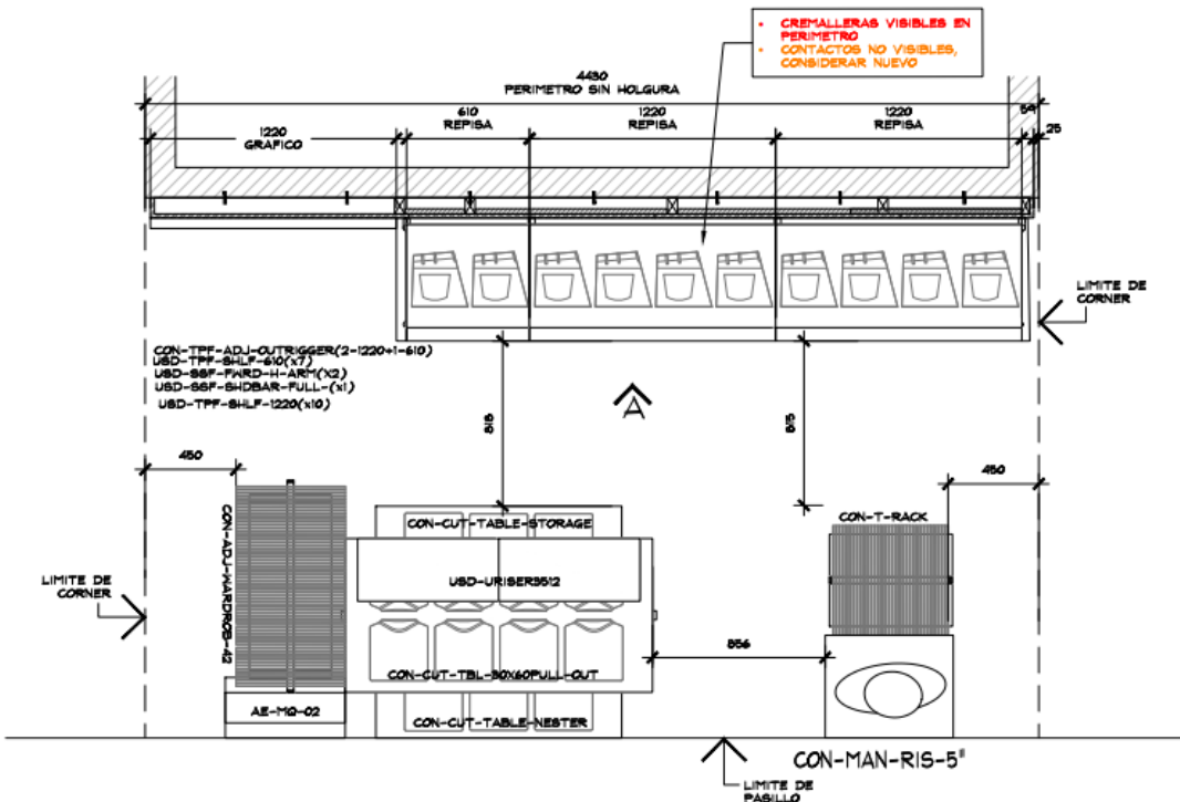
PLANTA DE MOBILIARIO ESC. 1:25
