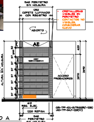
ALZADO A ESC. 1:50
