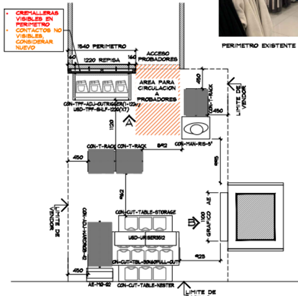
PLANTA MOBILIARIO ESC. 1:50
