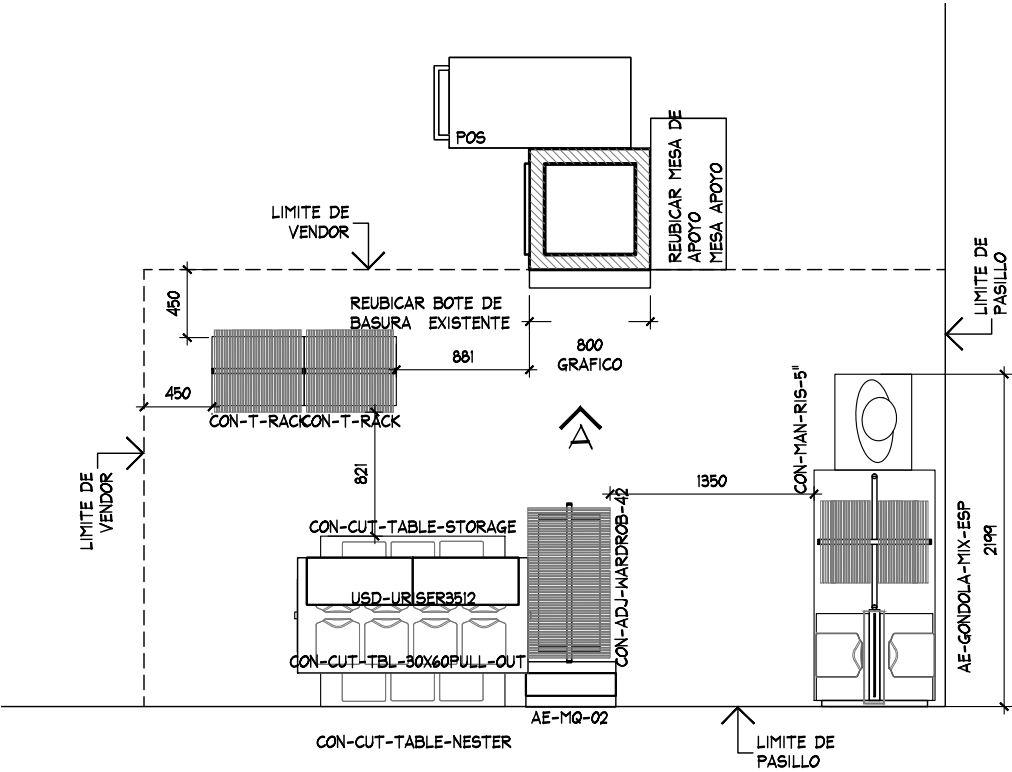
PERIMETRO EXISTENTE
