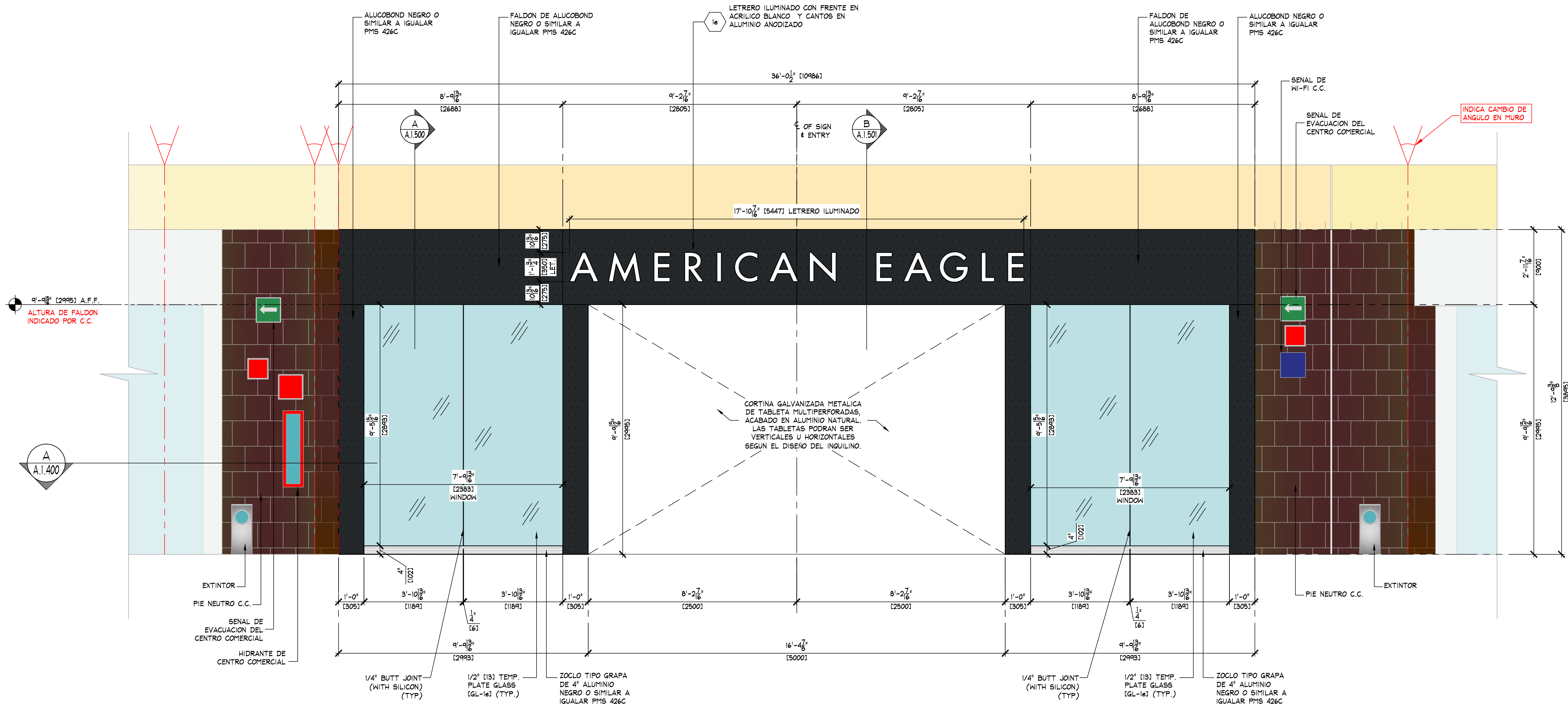
A STOREFRONT EXTERIOR ELEVATION A.1.300 SCALE: 1/2" = 1'-0" (1:25)
