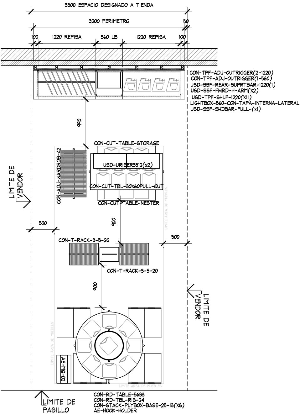
PLANTA GENERAL ESC. 1:50
